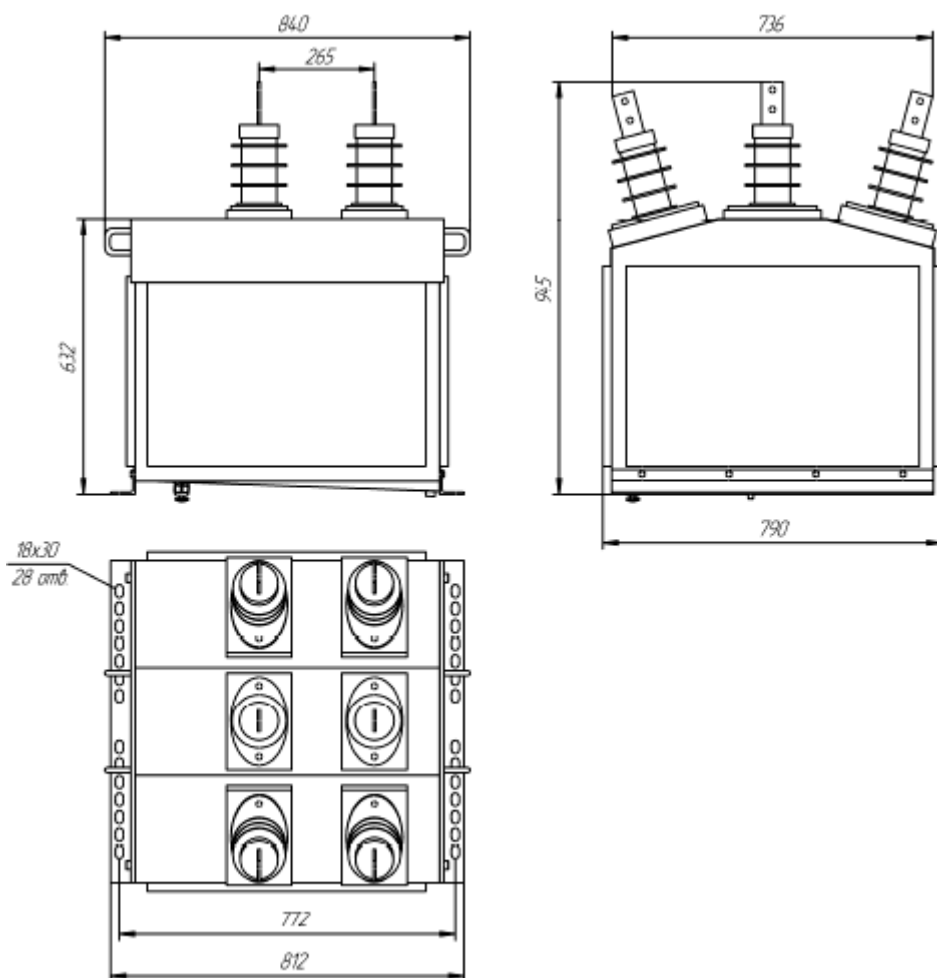
Рис. 9. Габаритные и установочные размеры коммутационного модуля
