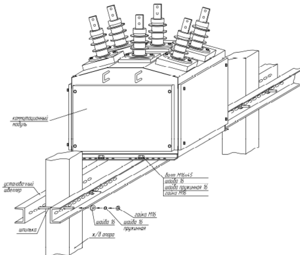
Рис. 12. Установка реклоузера на двух опорах
