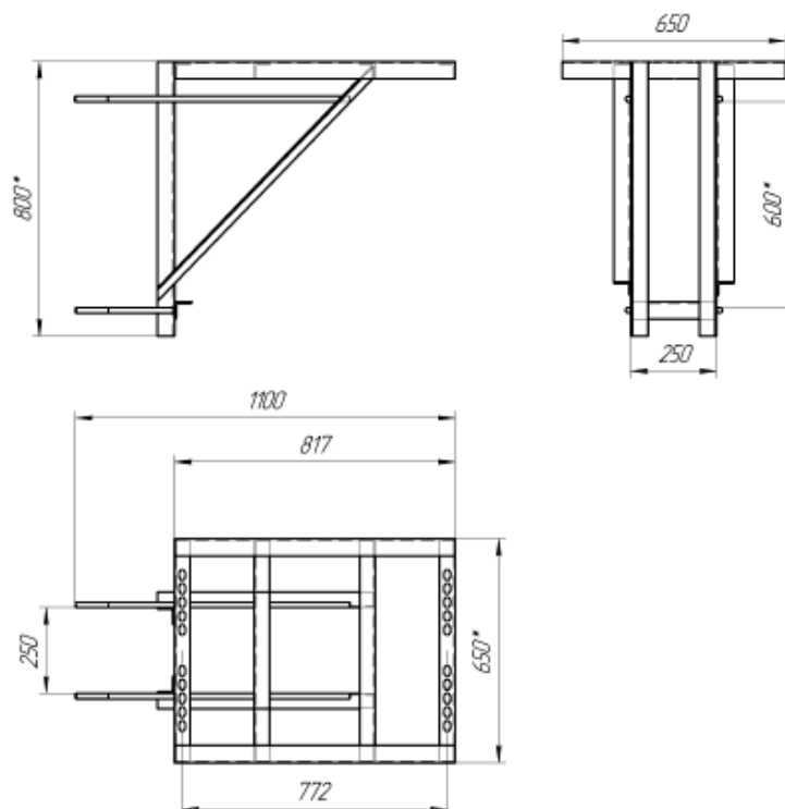
Рис. 11. Габаритные и установочные размеры монтажного комплекта для крепления на одну опору
