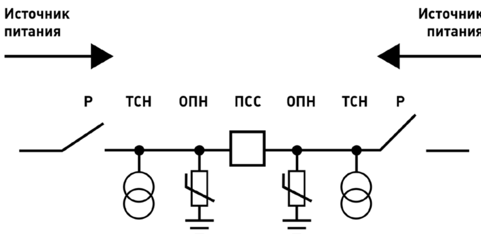
Рис. 2. Принципиальная схема включения реклоузера в линию при двухстороннем питании
