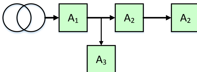
Рис. 3. Сеть с односторонним питанием
