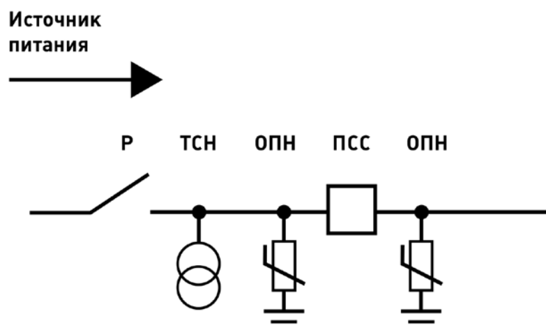
Рис. 1. Принципиальная схема включения реклоузера в линию при одностороннем питании
