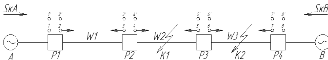
Рис. 5. Работа направленной защиты максимального тока.
