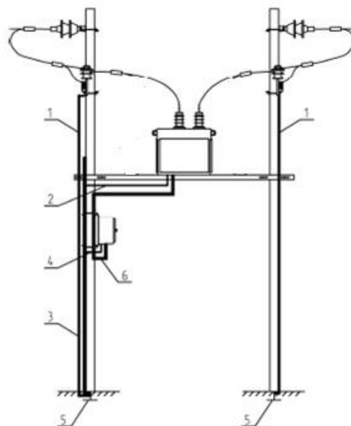
Рис. 8. Схема установки и заземления реклоузера на двух опорах
