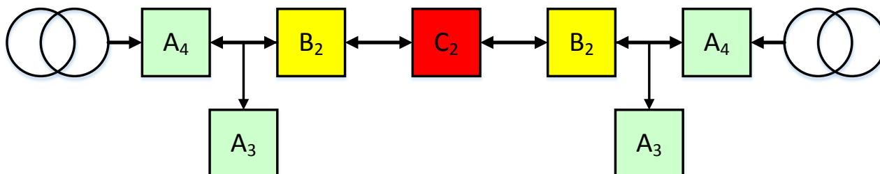
Рис. 4. Сеть с двусторонним питанием
