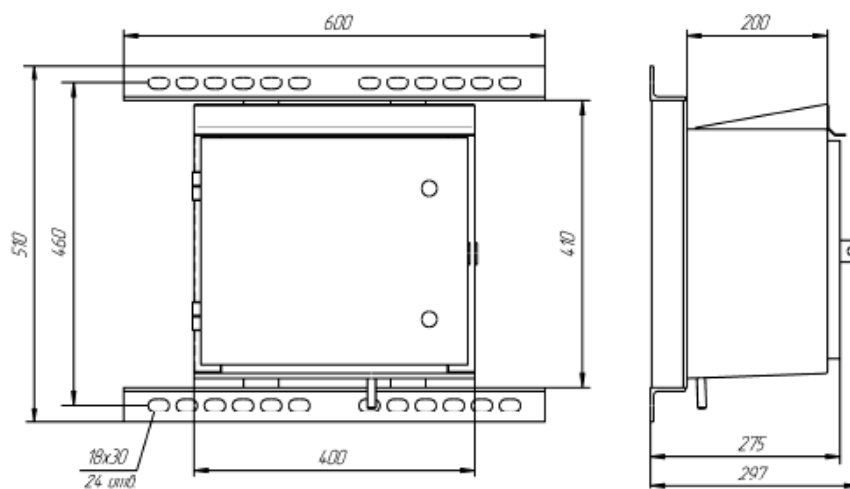
Рис. 10. Габаритные и установочные размеры шкафа управления
