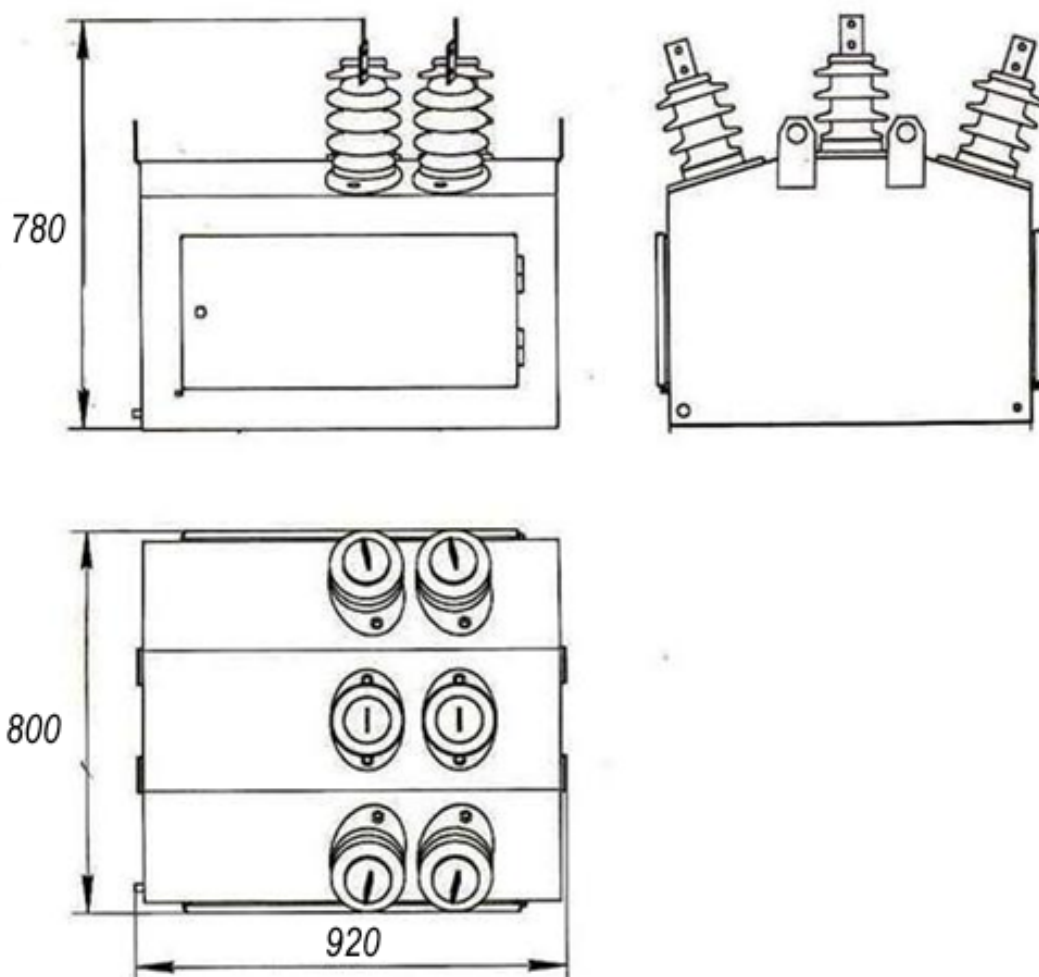
Рис. 1. Высоковольтный шкаф. Общий вид и габаритные размеры
