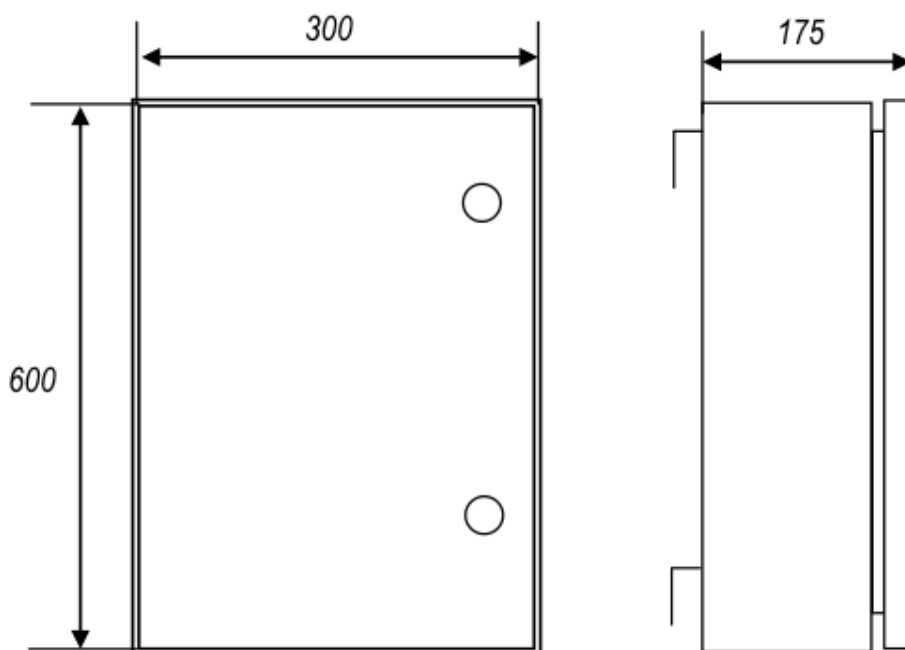
Рис. 3. Шкаф учета и передачи данных. Общий вид и габаритные размеры
